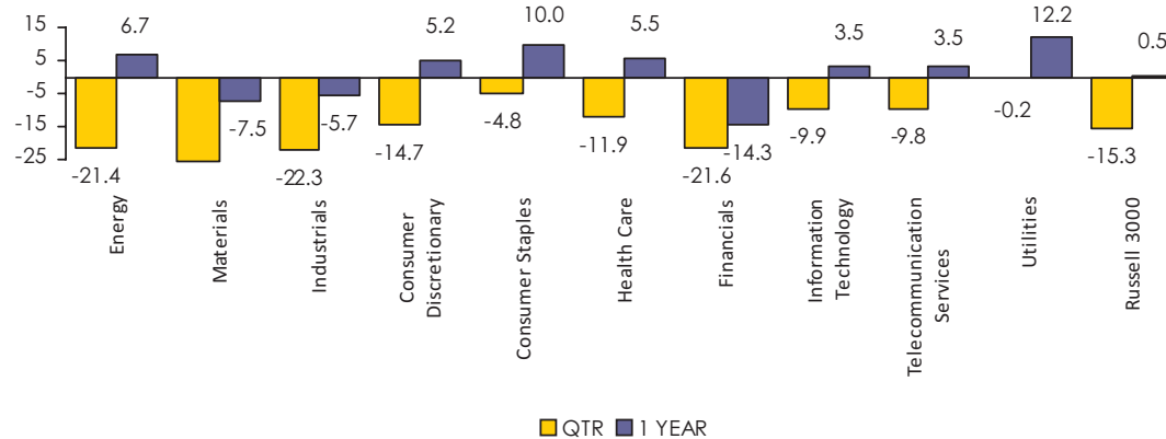
Sector Returns (%)
